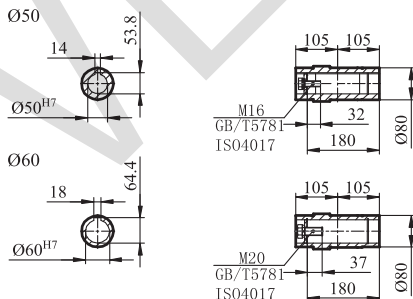
GSA/GSAZ/GSAF77输出轴
