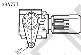
GSA/GSAZ/GSAF77输出轴
